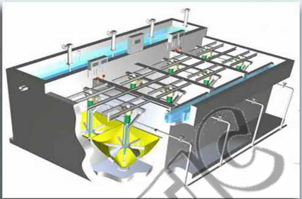
Instalasi CSF dalam bak beton
